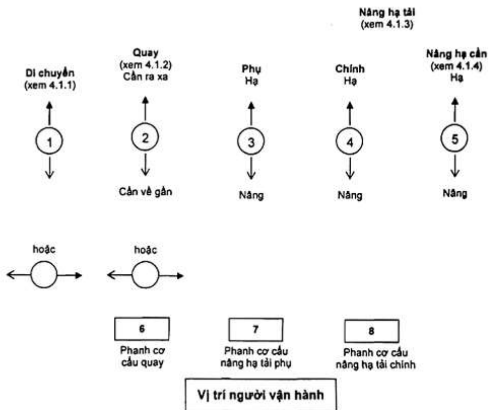
Hình 1 - Sơ đồ điều khiển cần trục có chiều dài cần cố định hoặc cần khớp xoay điều khiển hai chiều
