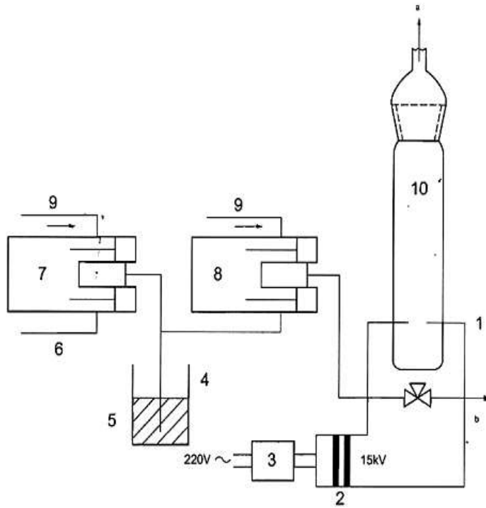
b) Thiết bị thích hợp cho việc thử nghiệm hỗn hợp khí
