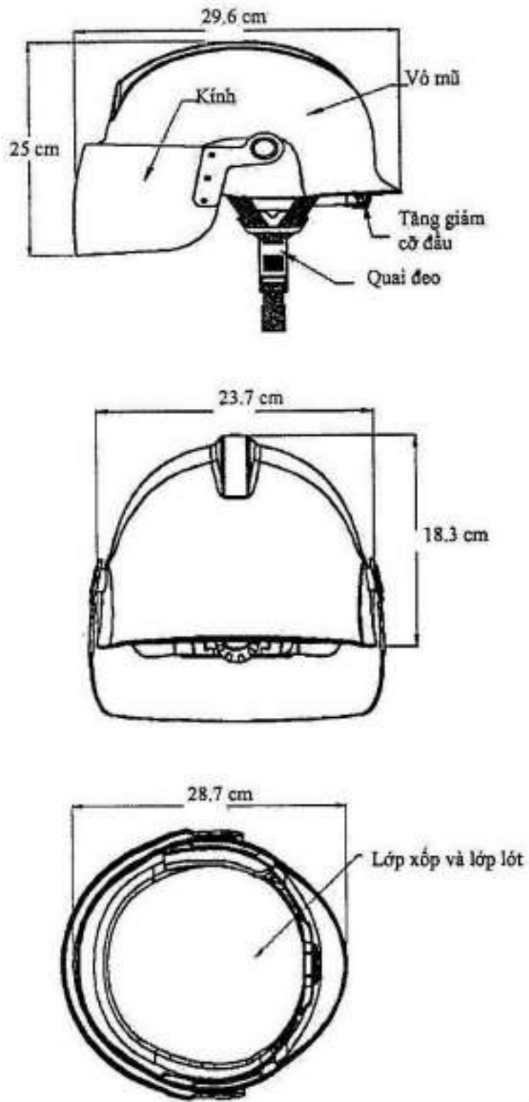
Chi tiết kỹ thuật mũ chữa cháy
